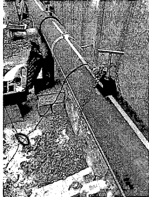
Misurazioni di portata con dispositivo ad ultrasuoni portatile del tipo clamp-on alla centrale di S. Filomena (strumentazione temporaneamente fornita dall'acquedotto di Acireale)
